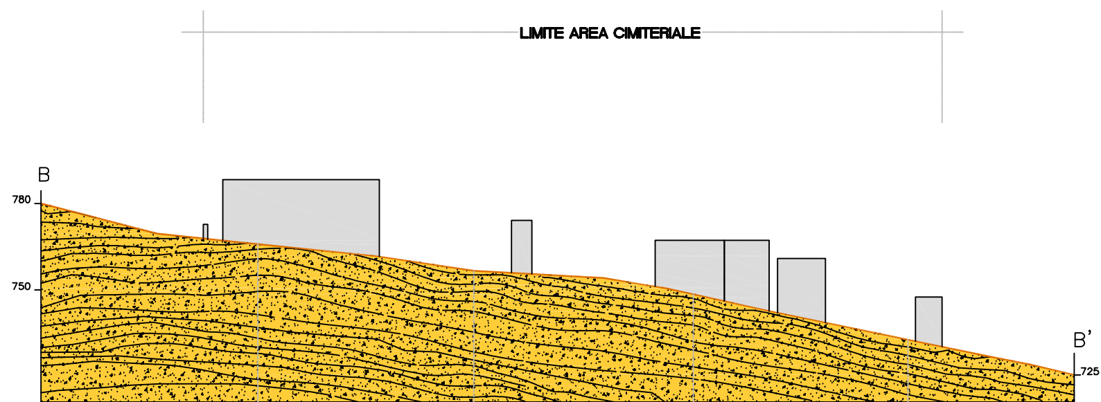
SEZIONE GEOLOGICA B-B'
